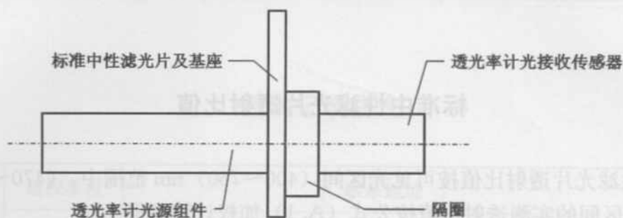
图1 示值误差校准示意图
