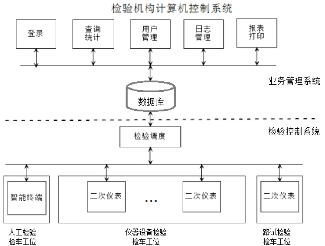
图 1 汽车检验机构计算机控制系统示意图
