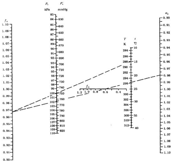
图 C3 非增压及机械增压柴油机功率校正系数图
