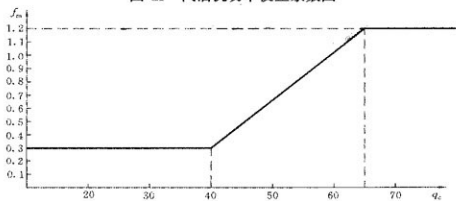
图 C2 f_m 与 q_c 的关系图
