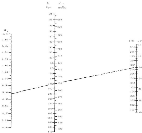
图 C1 汽油机功率校正系数
